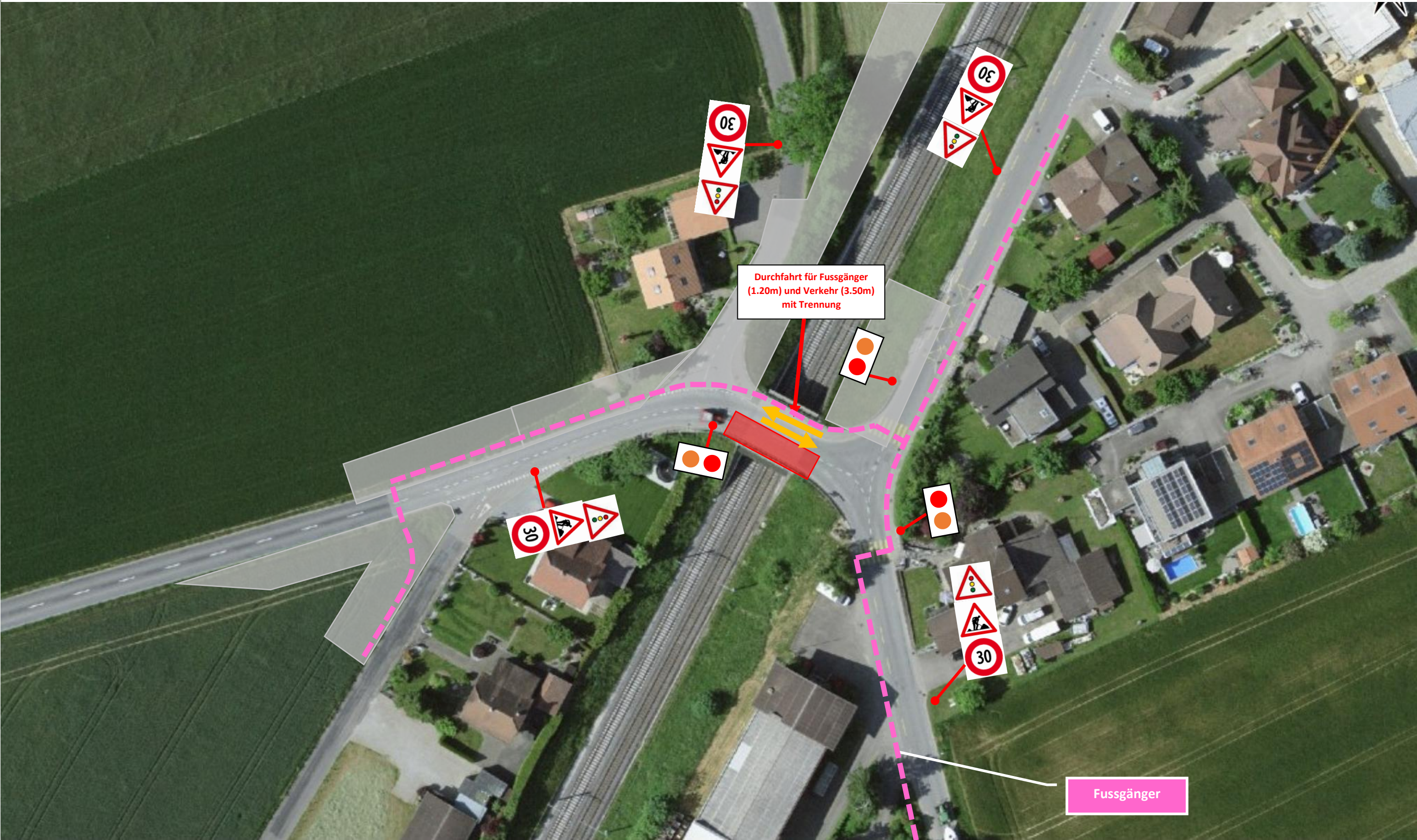
Detail 1 : Kreuzung Zelgmoosweg – Räschstrasse
